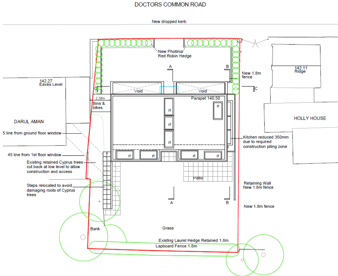
1:200 SITE PLAN
